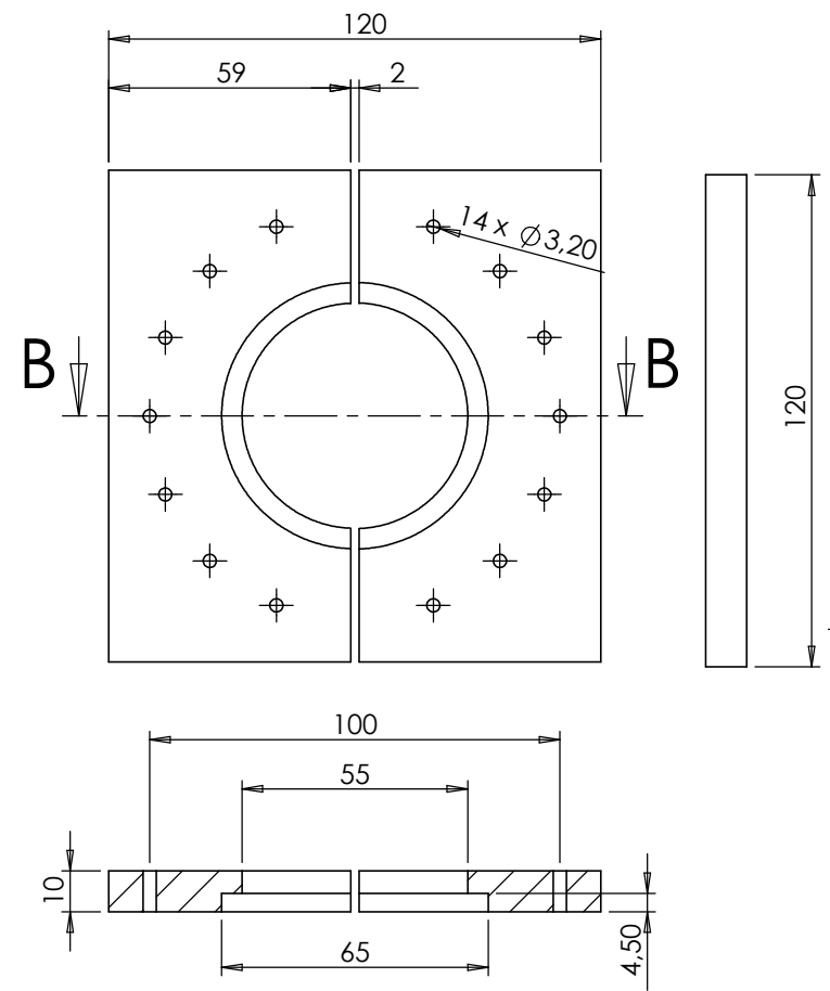
ŘEZ B-B MĚŘITKO 1 : 2
