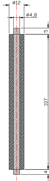
Vnitrek Koax. Kabelu.
