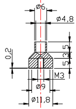
Matice ladiciho Terciku. Material: Cu
