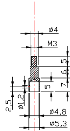
Redukce stredni vodic - konektor. Material: MS
