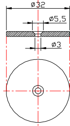
Vazebni tencik Material: Al nebo Cu. Lesteno.
